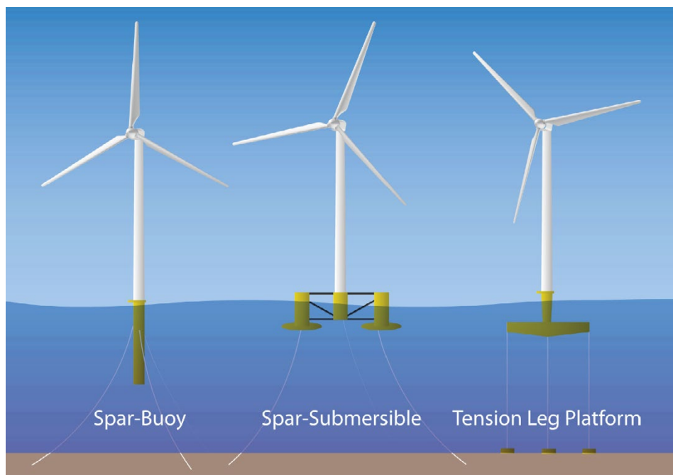
Figur 5. Olika typer av flytande vindkraftverk: Sparfundament, Spar-submersible och Tension leg platform .
